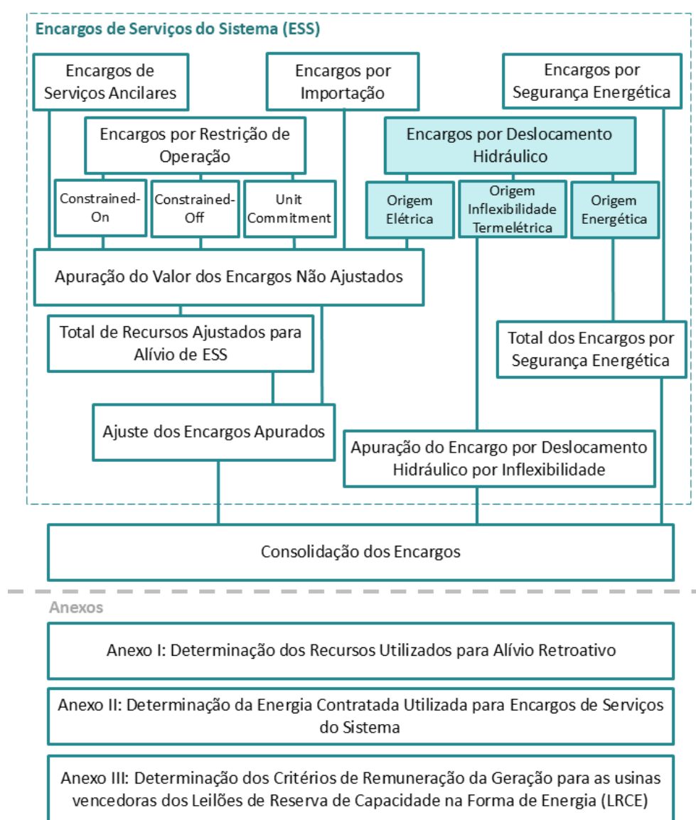
Figura 14: Esquema Geral do Módulo de Regras: "Encargos"
