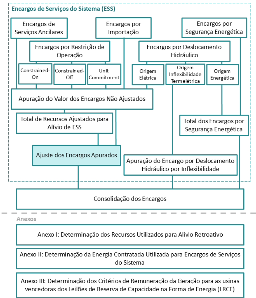
Figura 18: Esquema Geral do Módulo de Regras: “Encargos”
