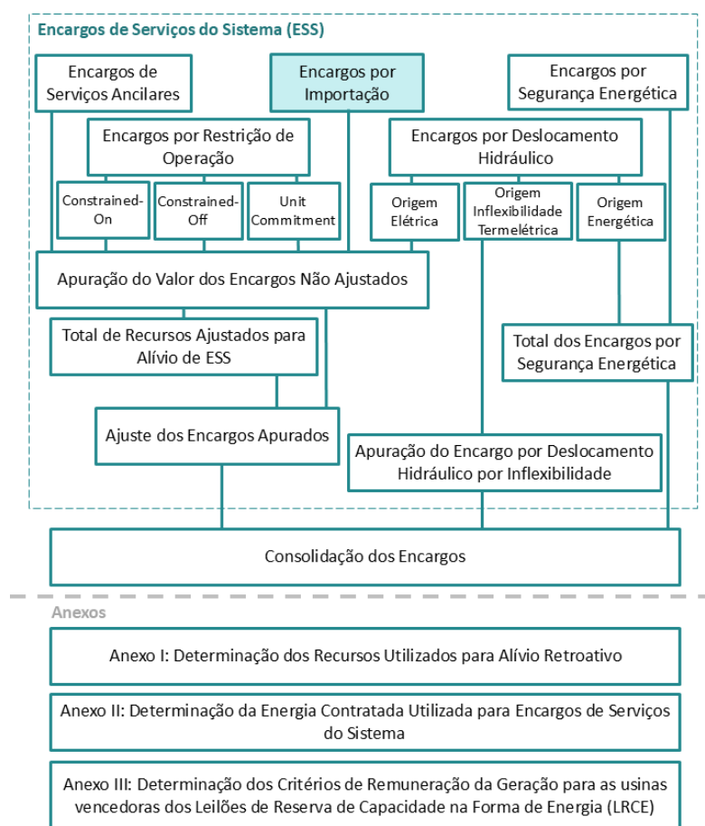
Figura 12: Esquema Geral do Módulo de Regras: "Encargos"
