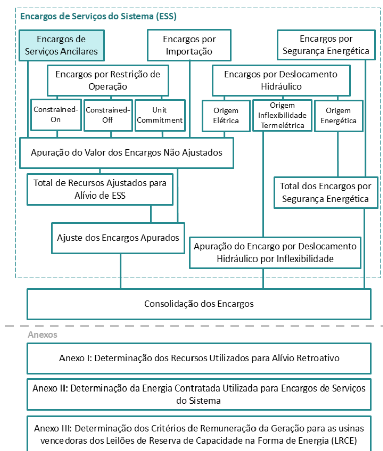
Figura 11: Esquema Geral do Módulo de Regras: “Encargos”
